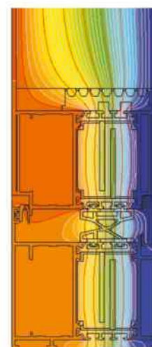
przykładowy rozkład izoterm dla złożenia ościeżnicy i skrzydła drzwiowego systemu PD GN 75
